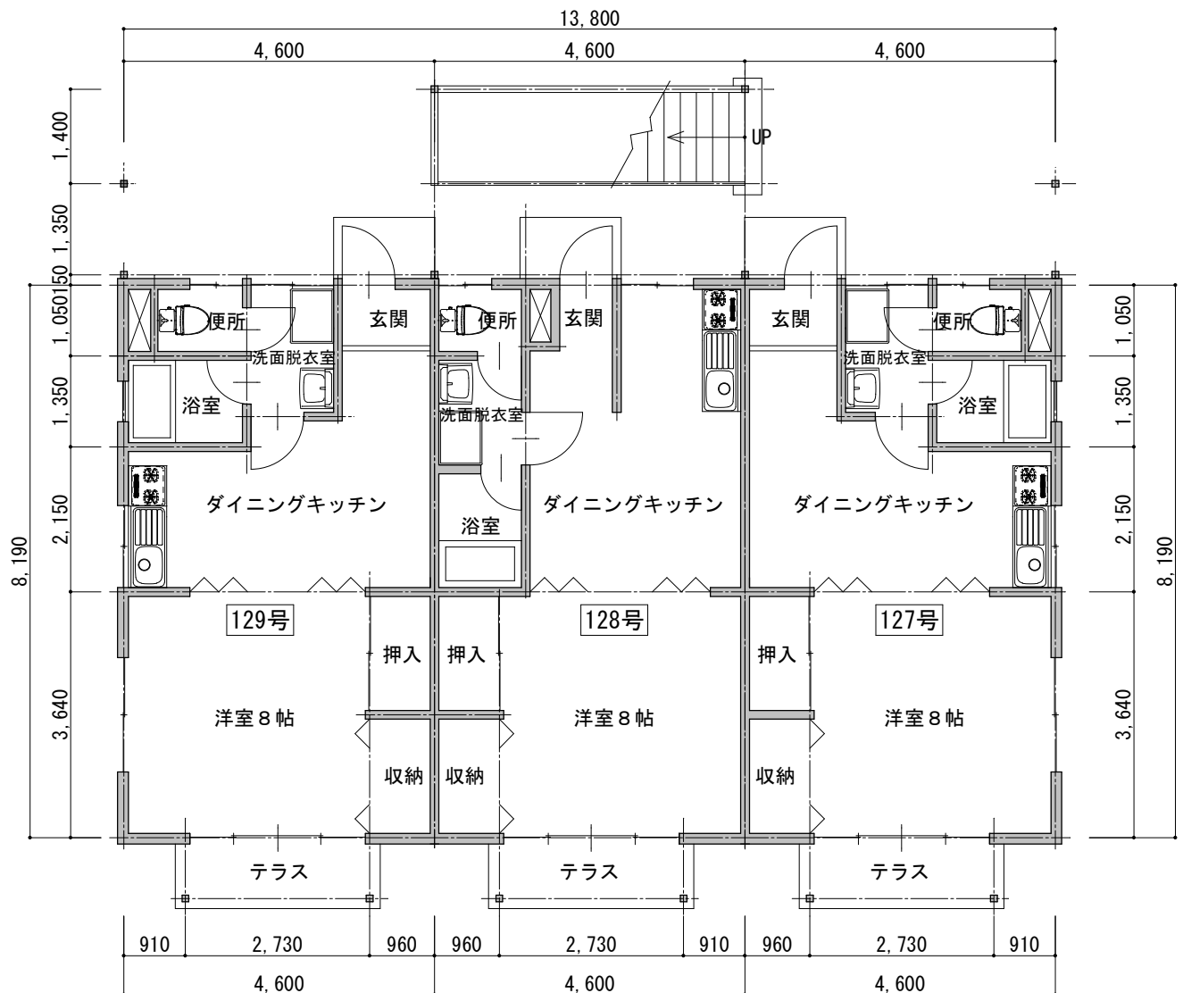
1階平面図
