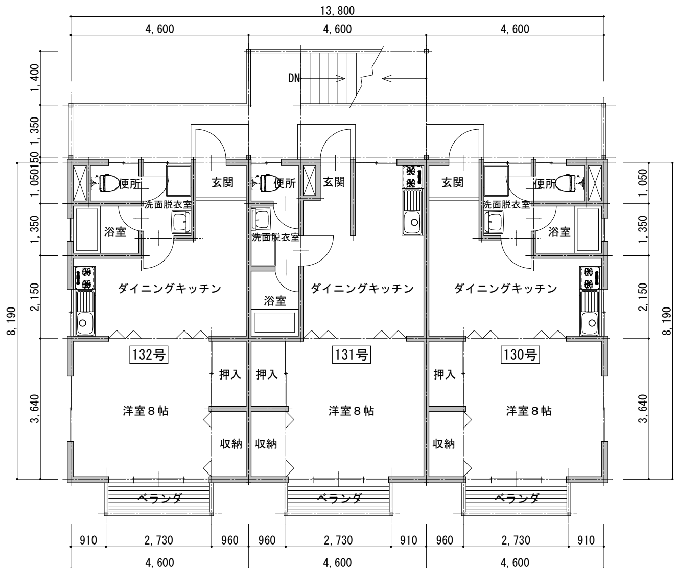
2階平面図
