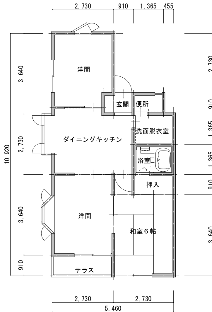
2階平面図
