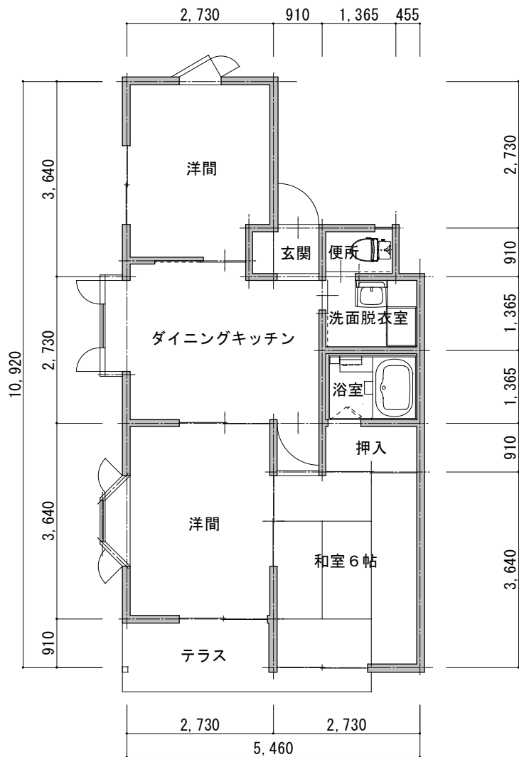
1階平面図
