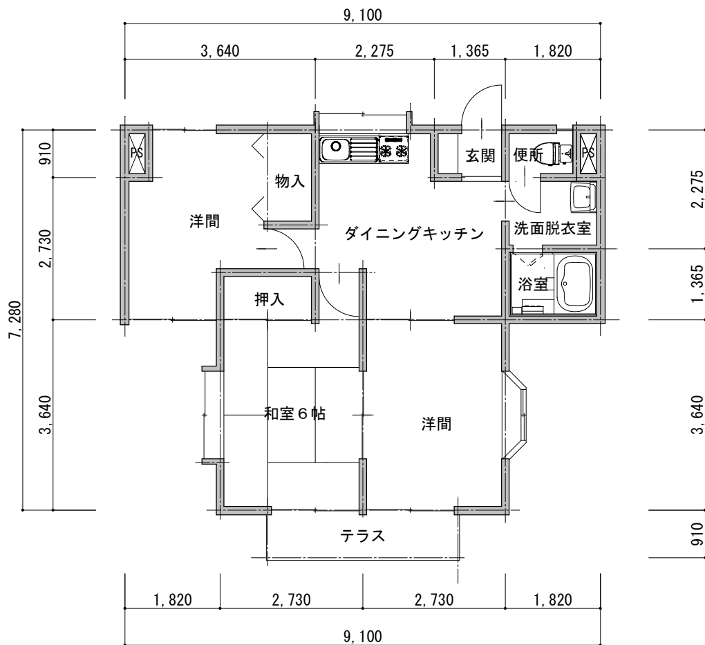
平面図
