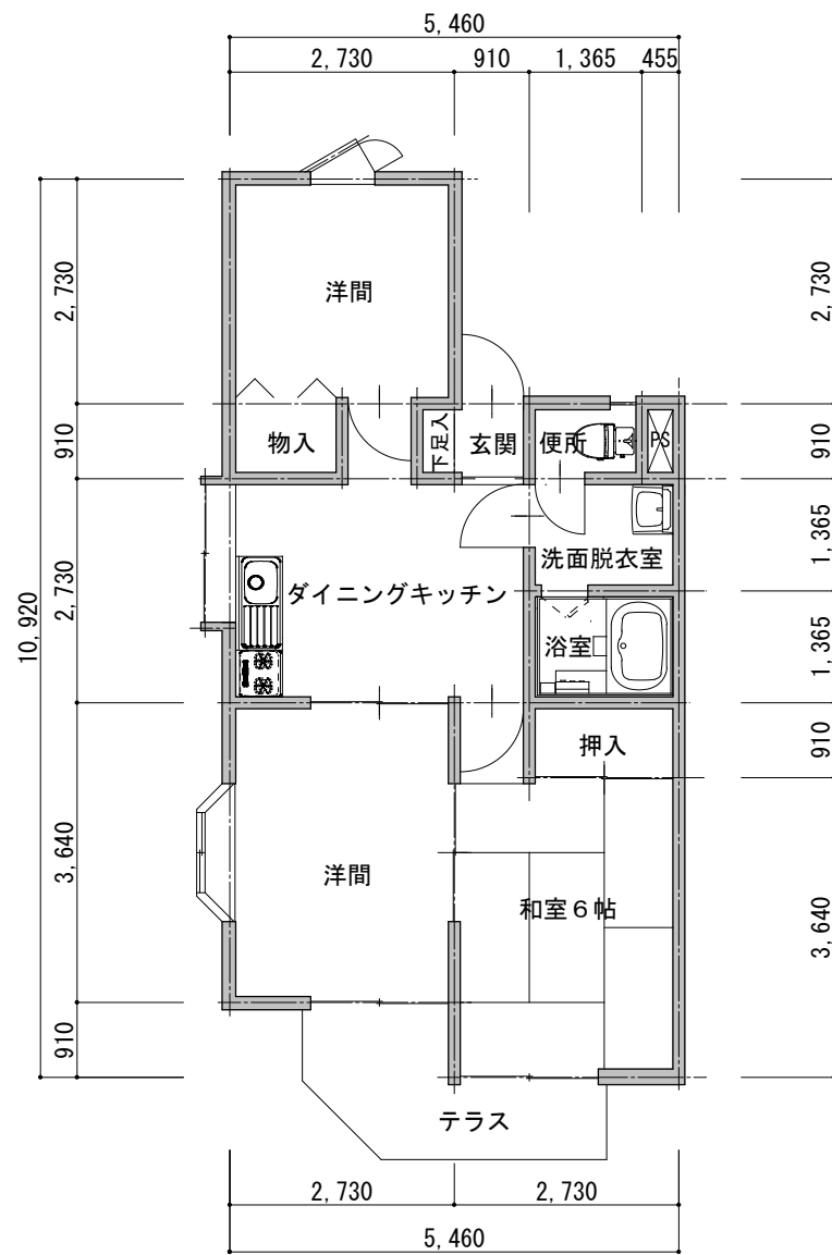
平面図
