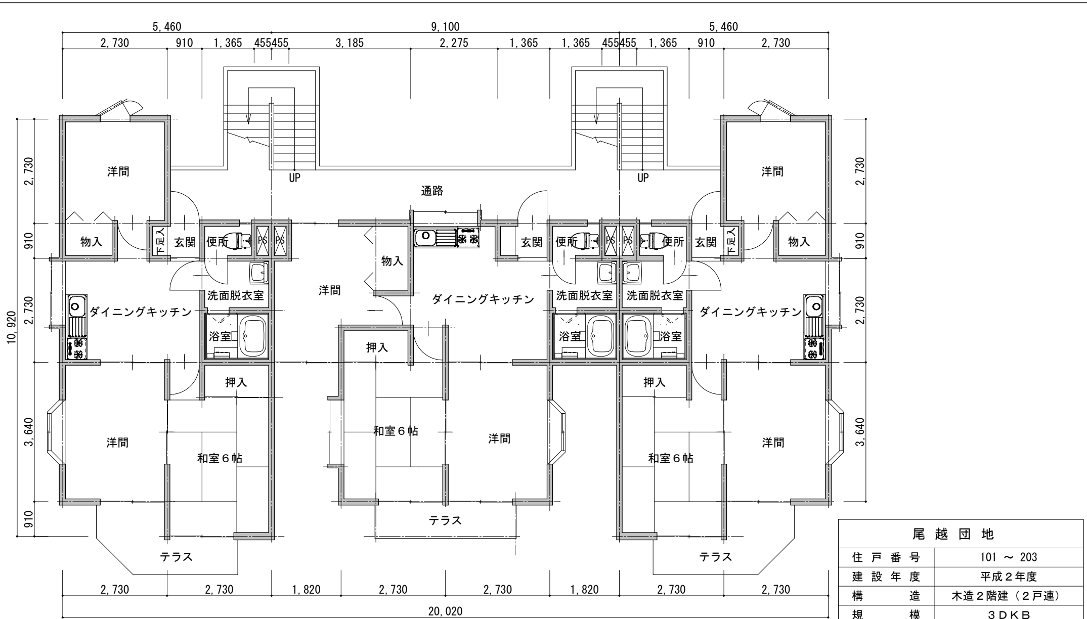
1階平面図
