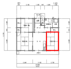
平面図
