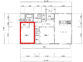
平面図
