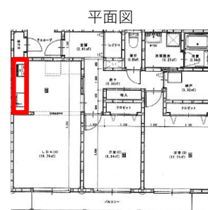
キッチン
